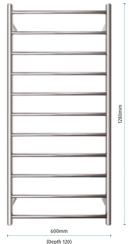
Forme 11 bar ROUND HTR-TR1101M
